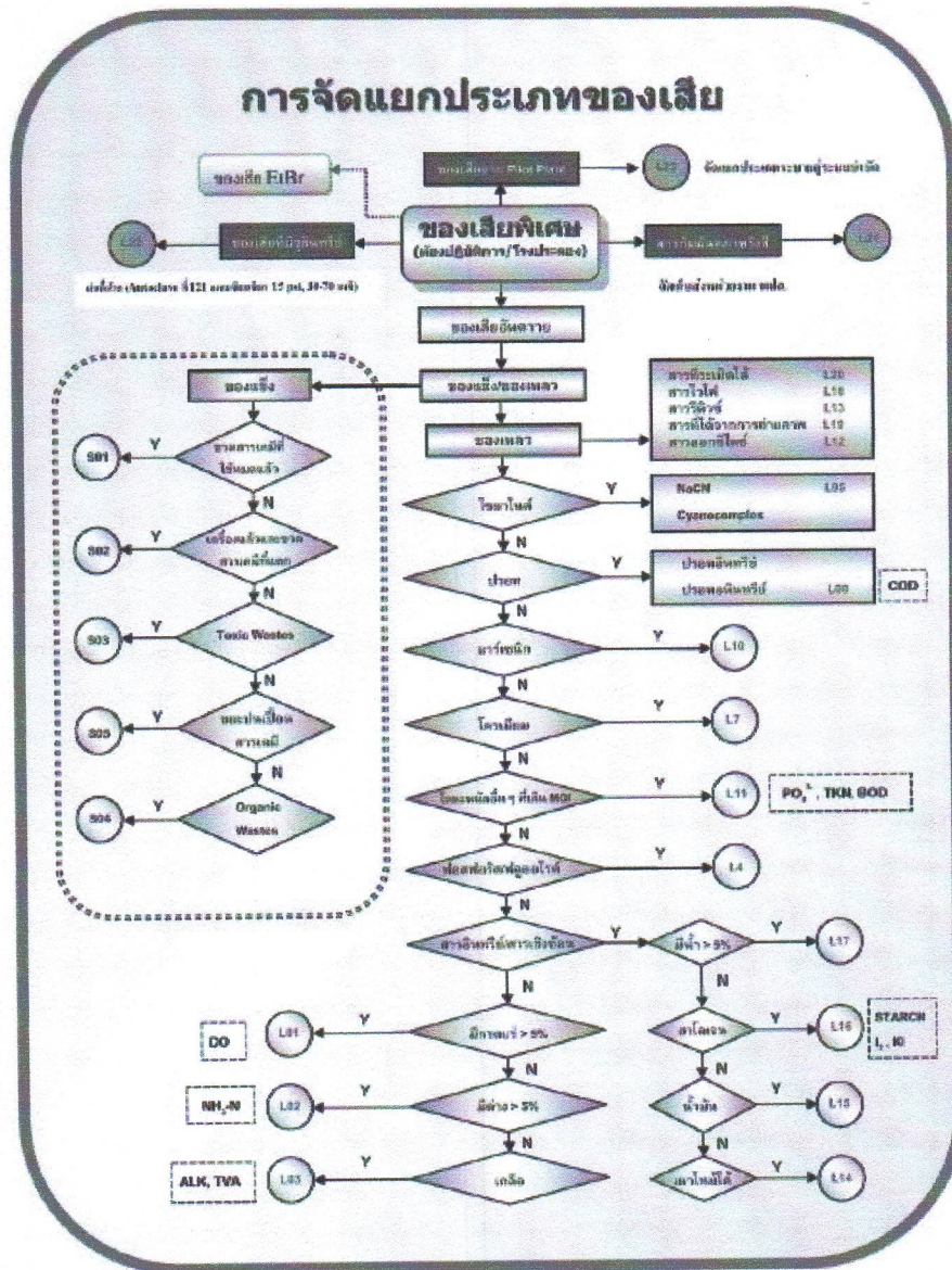
5. Flow chart แสดงการจัดจำแนกประเภทของเสียอันตราย (ของแข็ง 5 ประเภท, ของเหลว 18 ประเภท และของเสียอันตรายพิเศษ 4 ประเภท)
